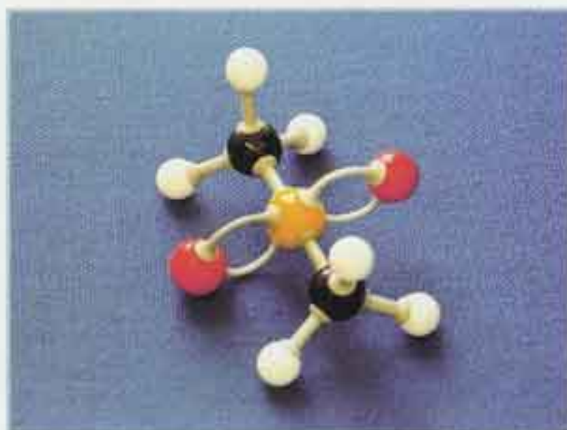
Amarillo = S ; Rojo = O ; Negro = C ; Blanco = H
